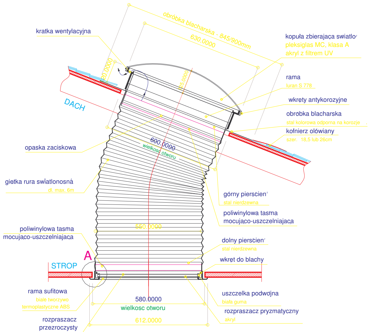
Schemat zestawieniowy elementów świetlika rurowego maxiSolar® big
